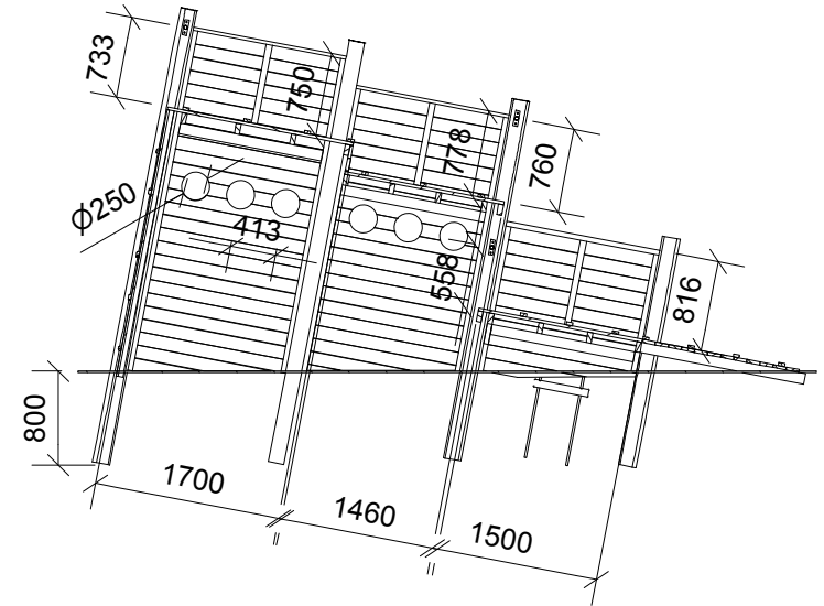
A-A (1:75)
